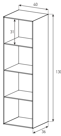
OP85V (vertical) OP85H (horizontal)
